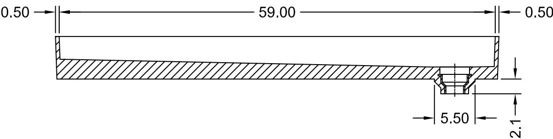
SECTION A-A
